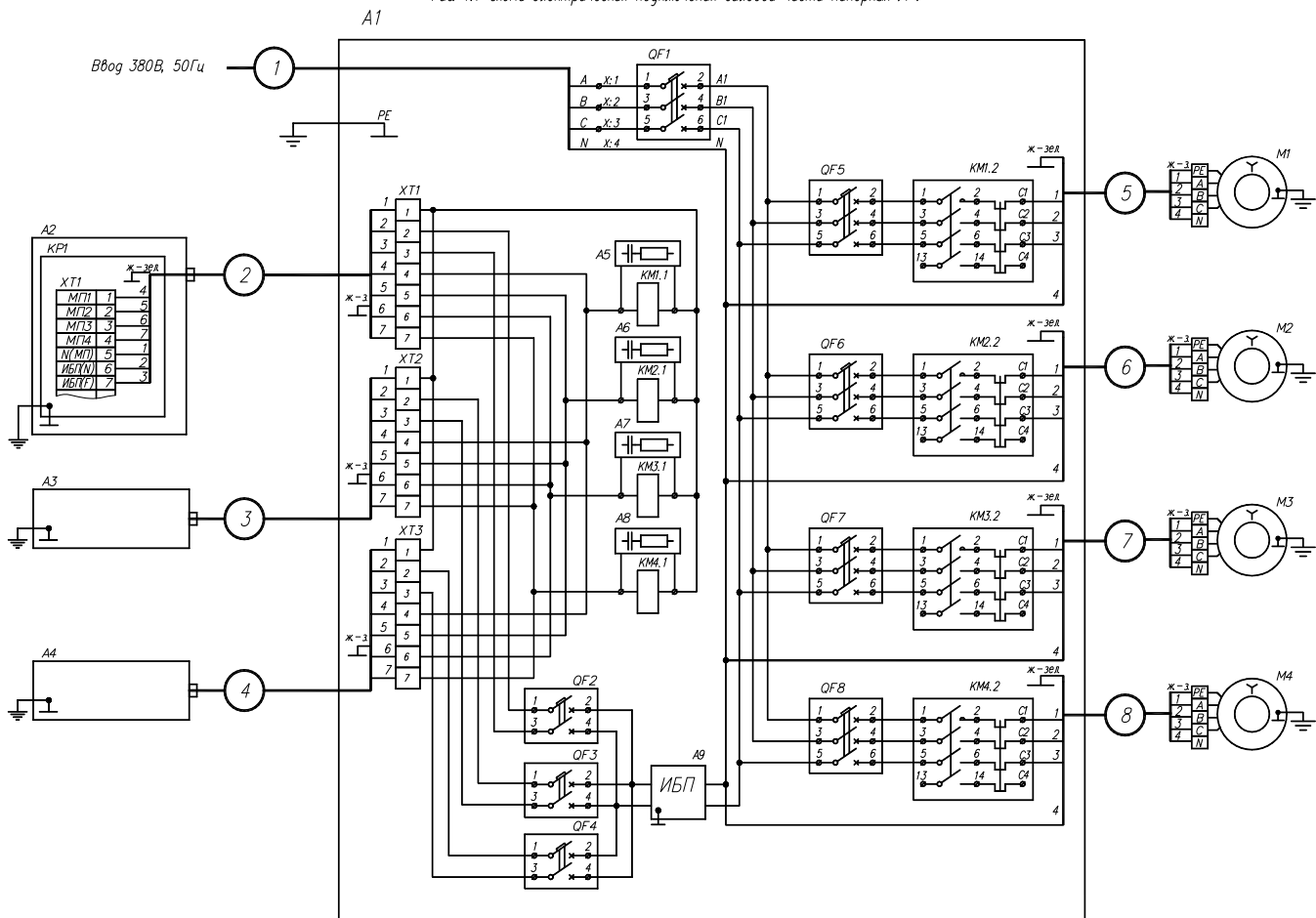
Рис. 1.1 Схема электрическая подключения силовой части напорных УТ.
