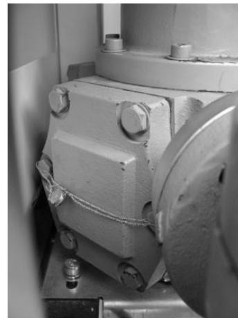
Рисунок В.2 Пломбировка измерителя объёма
