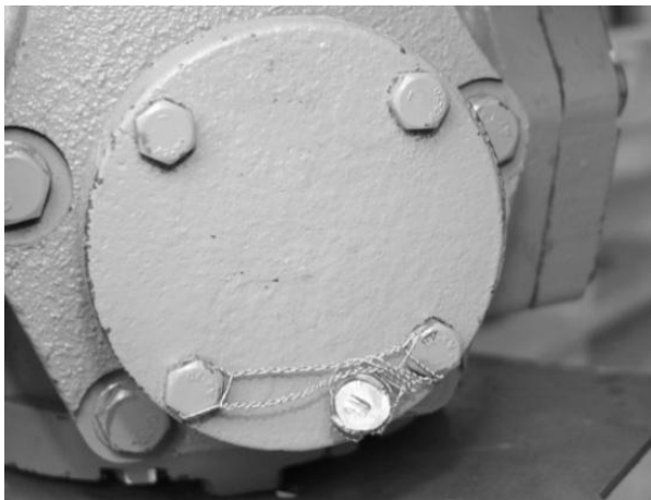
Рисунок В.2 Пломбировка измерителя объёма
